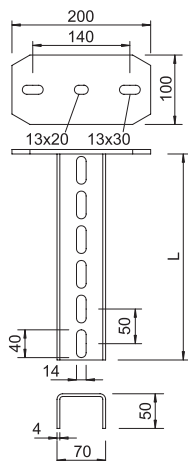
Abmessungen
