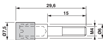
Maßzeichnung
