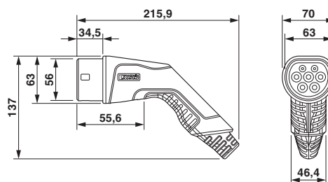
Maßzeichnung Fahrzeug-Ladestecker
