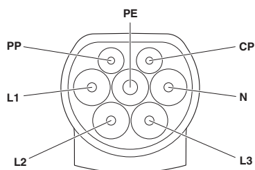
Pinbelegung Infrastruktur-Ladestecker
