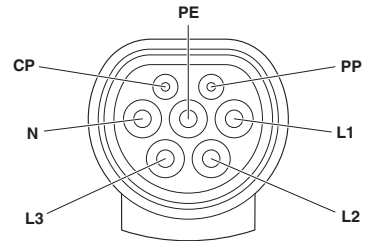
Pinbelegung Fahrzeug-Ladestecker
