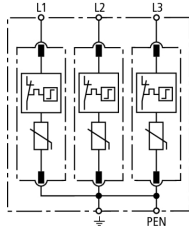
Prinzipialschaltbild DG M TNC 440
