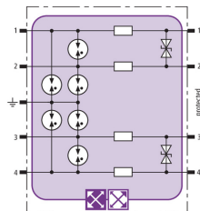
Prinzipialschaltbild BXT ML4 BD EX 24
