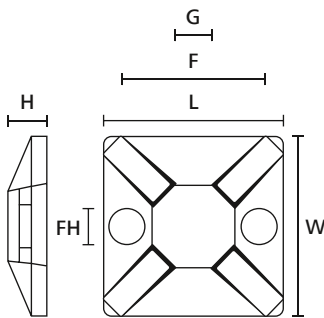
MCMB Sockel (Seitenansicht und Draufsicht)
