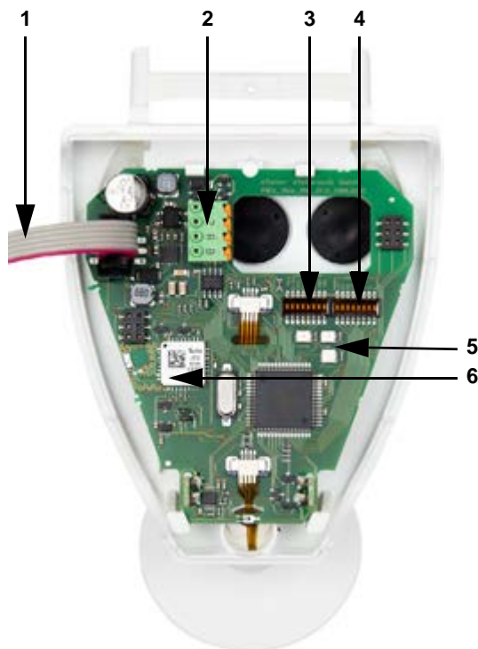
Abb. 12: Übersicht Platine
