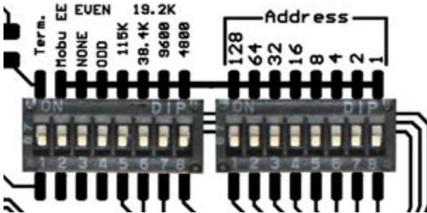
Abb. 13: Detailsicht Dipschalter
