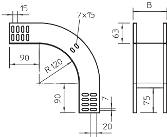
Abmessungen
