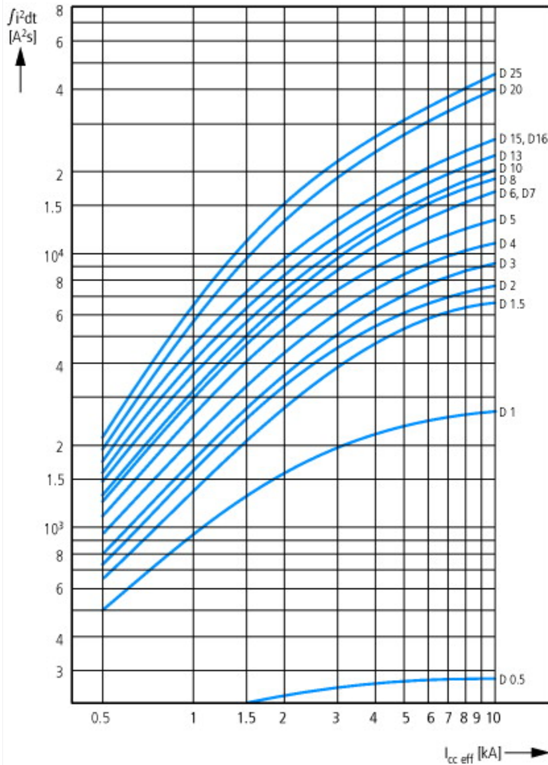
Durchlassenergie \int i^2 dt Charakteristik D (0,5 - 20 A), 277 V
