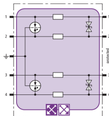
Prinzip Schaltbild BXT ML4 BD 60
