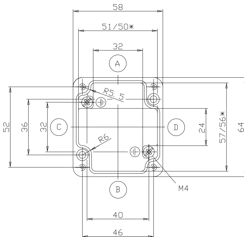
UNTERTEIL
