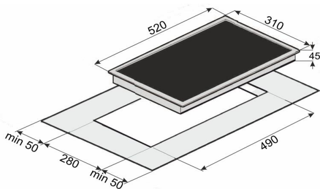
Einbauskizze
