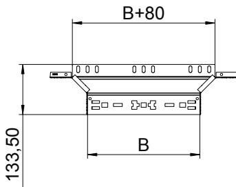
Abmessungen
