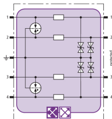
Prinzipschaltbild BXT ML4 BE 60
