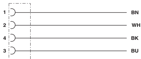
Kontaktbelegung der M12-Buchse
