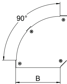
Abmessungen
