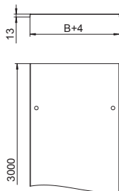
Abmessungen
