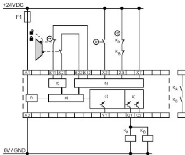
Schaltungsbeispiel
