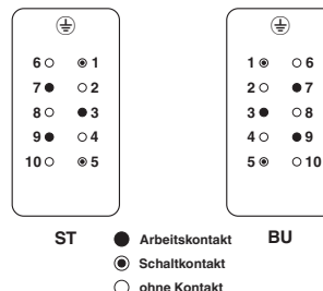
Schemazeichnung
