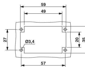
Maßzeichnung
