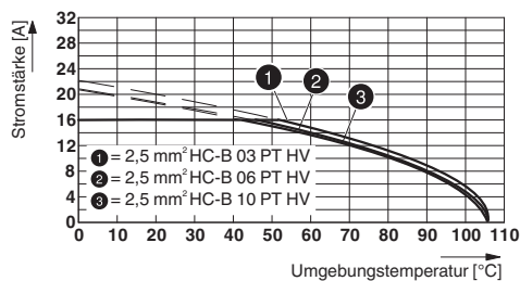
Derating-Diagramm für 2,5 mm²
