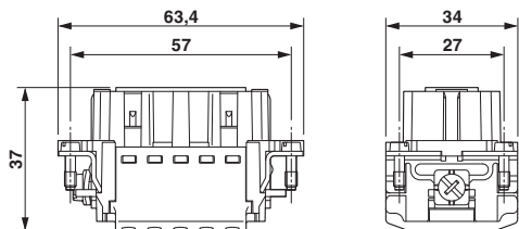
Maßzeichnung
