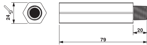
Maßzeichnung
