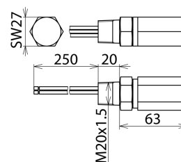
Maßbild DPI CD EXD 230 24 M
