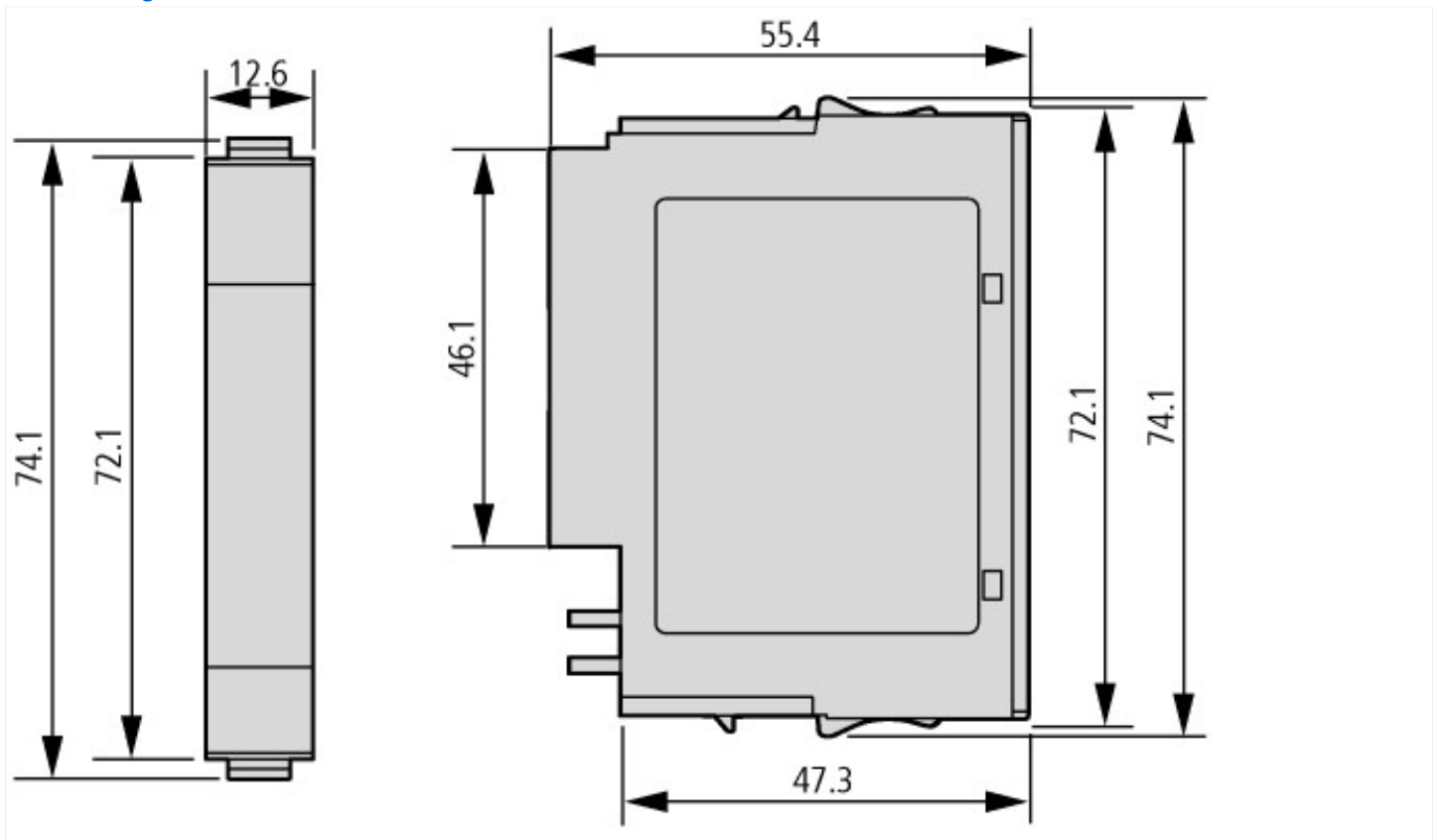
Abmessungen
